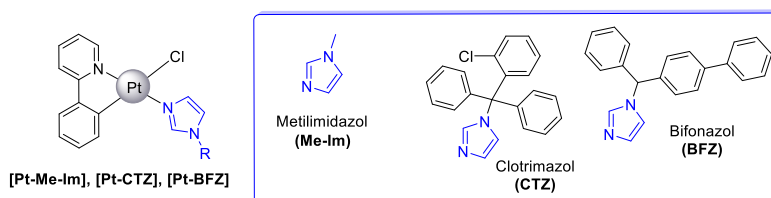
Fig. 1. Complejos ciclometalados de Pt(II) con ligandos derivados de imidazol.
